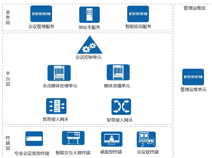
图1 智慧会议系统技术框架
